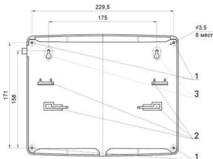
Рисунок 4 – Установочные размеры
