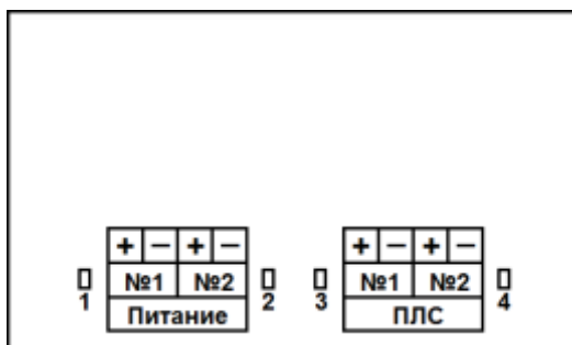
Рисунок 13 – Назначение клемм
