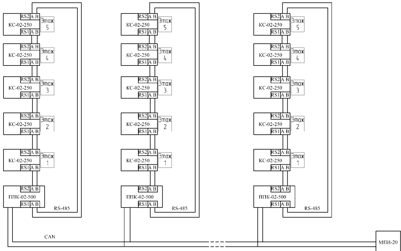
Рисунок 7 – Схема организации интерфейса RS-485
