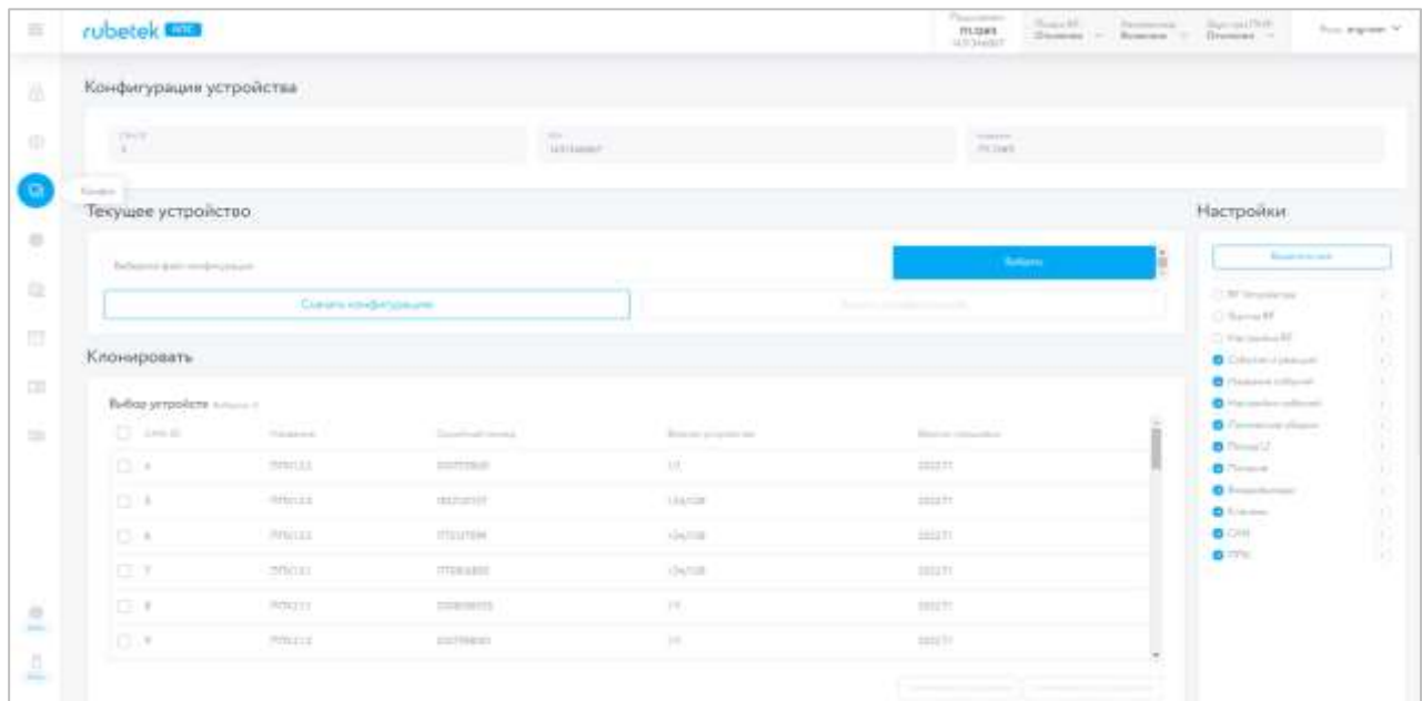
Рисунок 24 – Выгрузка дампа
